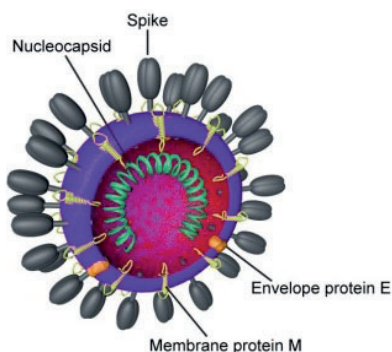
· Obrázek 1. · Schéma struktury virionů COVID-19 znázorňující hroty, které tvoří "korunu" (sluneční koruna - odvození názvu)
